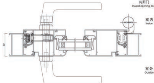
内开门
