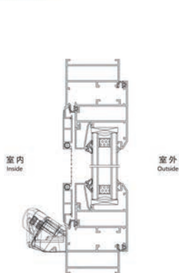
五金装配图
