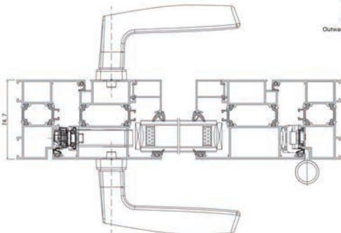
五金装配图
