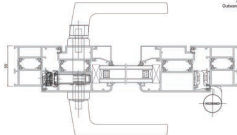
外开门
