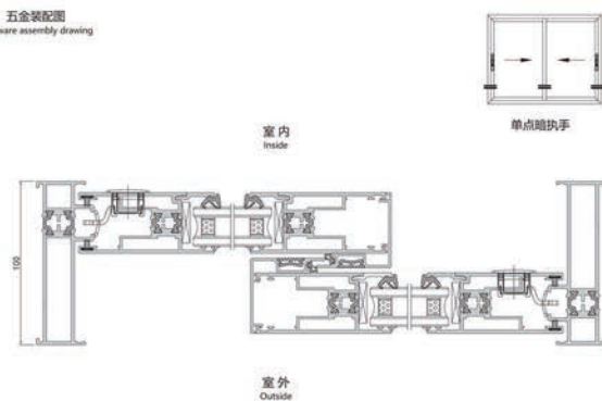
五金装配图
