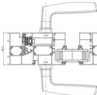
五金装配图
