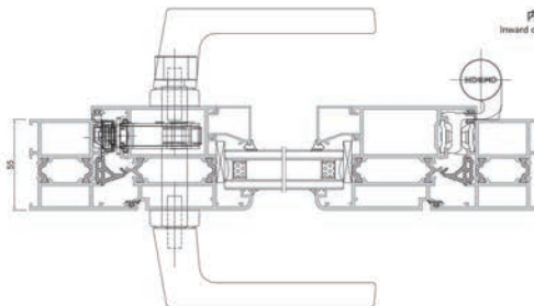
内开门
