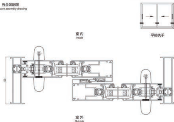
五金装配图
