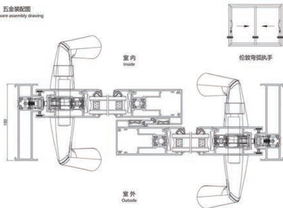
五金装配图
