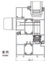
外悬窗
