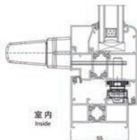
外悬窗
