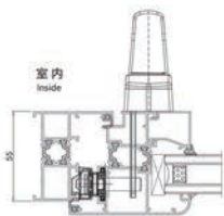
外开窗
