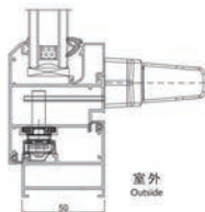
外悬窗
